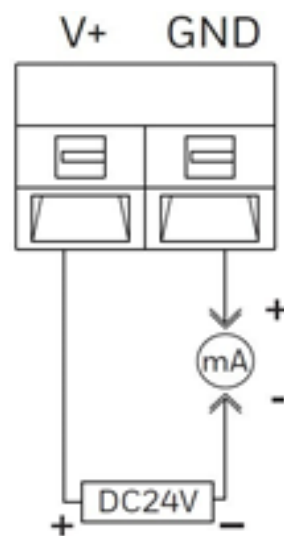
4-20mA
