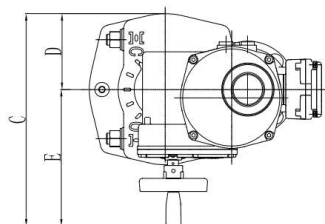
NOM16(25)H2000P(B)/NOM16(25)H4000P/NOM16(25)H5000P
